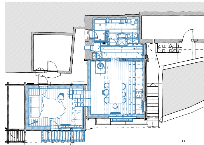
Plan rez-de-chaussée
