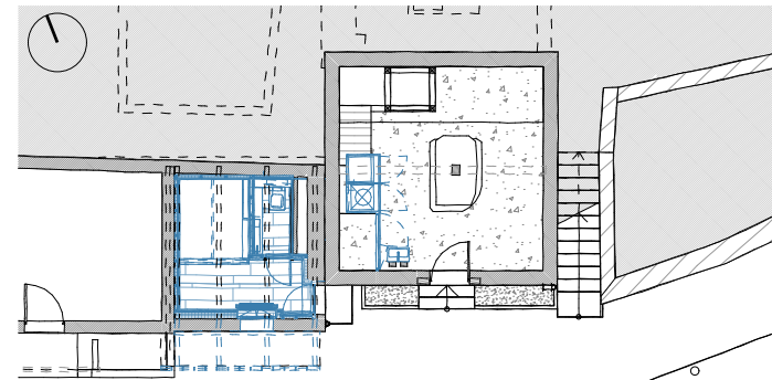
Plan sous-sol
