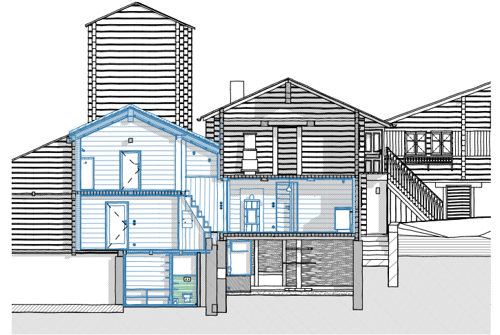
Coupe longitudinale
