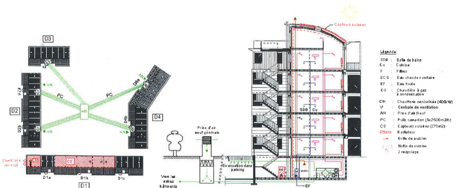
Schéma de principe chauffage + ventilation double flux
