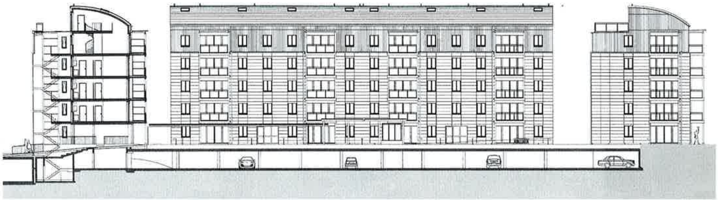
Coupe sur immeuble D2
