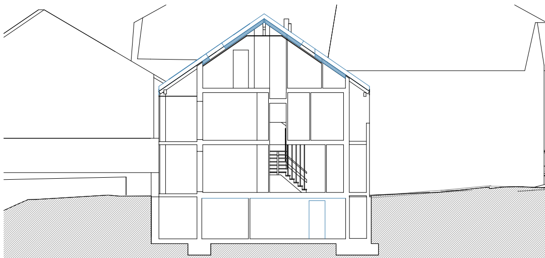
Coupe transversale
